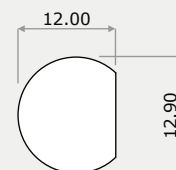
面板安裝孔尺寸
