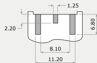
PCB板焊接建議圖 ■
