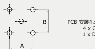
PCB板安裝孔尺寸
