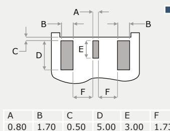
PCB板焊接建議圖
